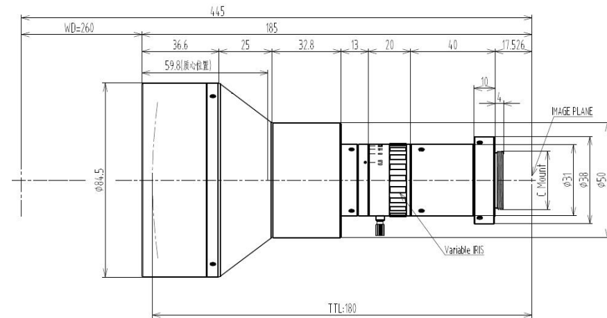
SNT1IR027W260C-I
